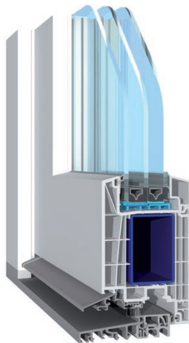
Schnittdarstellung, schematisch
